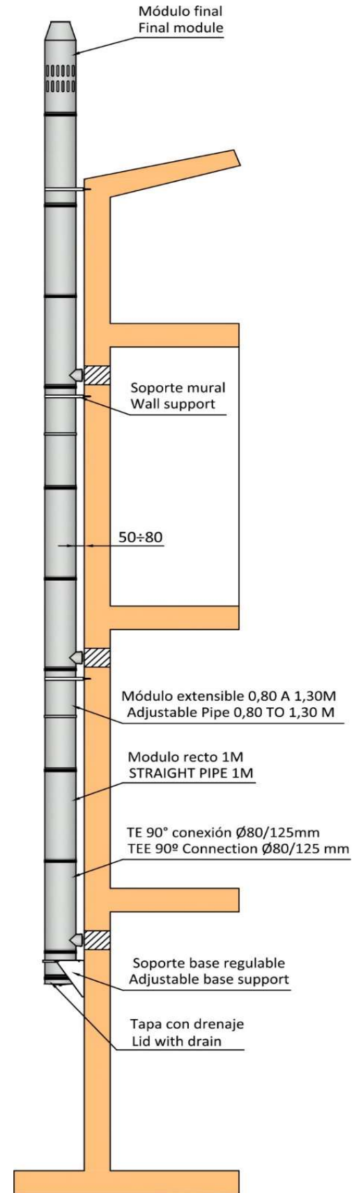
Ejemplo de montaje para 3 calderas
