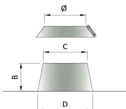
HICU CUBREAGUAS ALUMINIO 0-35° + COLLARÍN ANTILLUVIA ALUMINIUM FLASHING 0-35° + STORM COLLAR
