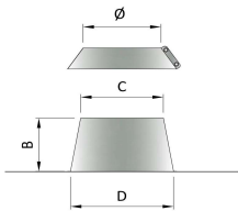
HICU CUBREAGUAS ALUMINIO 0-35° + COLLARÍN ANTILLUVIA ALUMINIUM FLASHING 0-35° + STORM COLLAR
