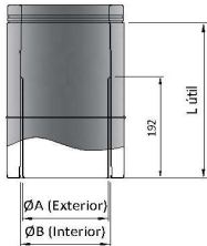
KWKVKT EXTENSIBLE VITRIFICADO A KW DE 0,33 m CONNECTING PIPE STARTER LENGHT 0,33 m
