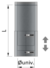
KWAR KW ADAPTADOR AJUSTABLE 0,5 m ADJUSTABLE CONNECTING PIPE 0,5 m
