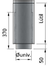
KWKVA EXTENSIBLE VITRIFICADO A KW DE 0,5 m CONNECTING PIPE STARTER LENGHT 0,5 m
